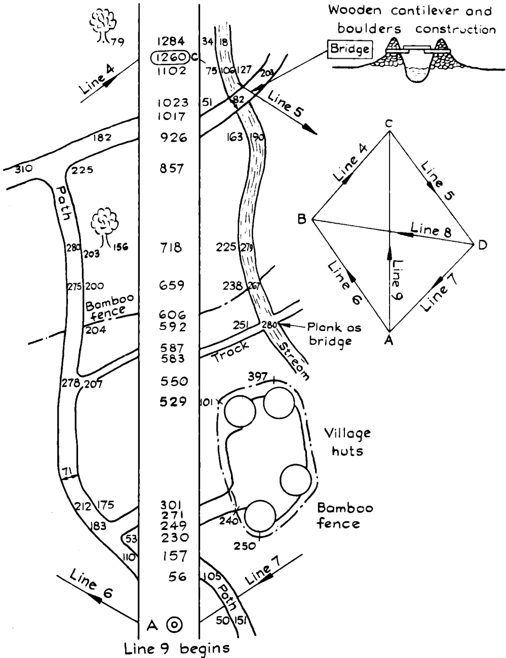
Fig. 8. A tape survey
